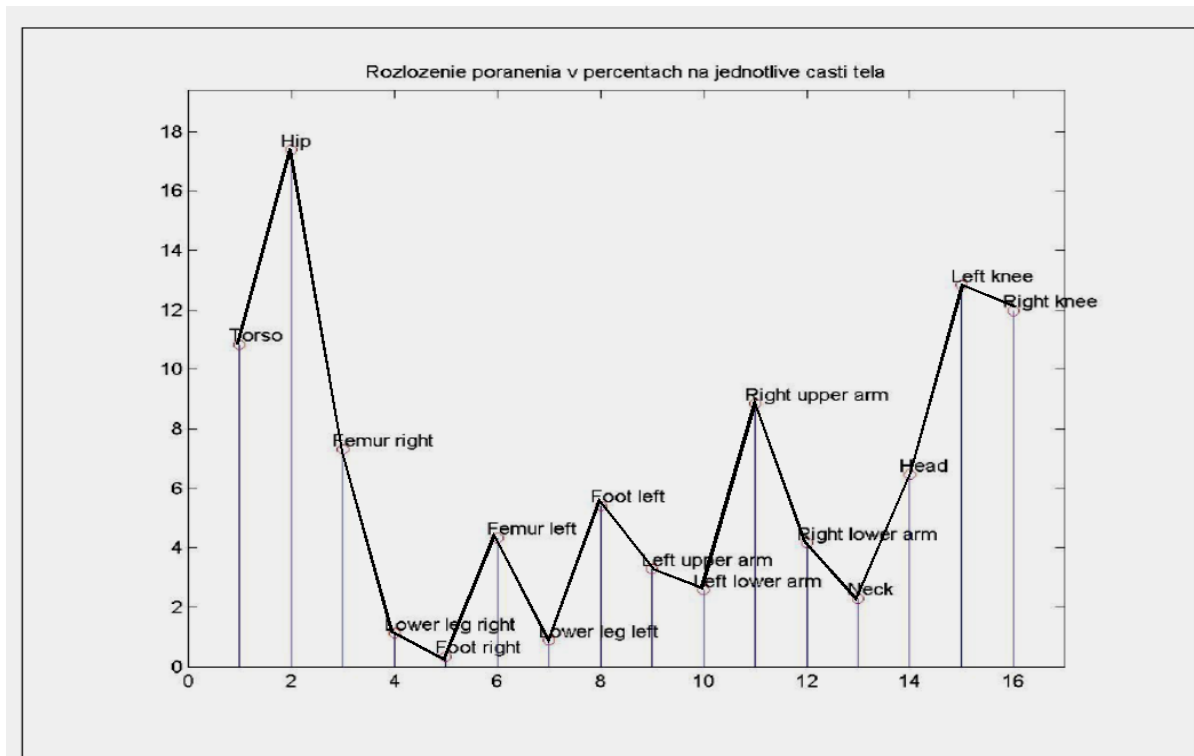
Obr. 10 Individuálna signatúra „Koefficienty kontaktov“ vypočítaná z PC Crash pre jednotlivé časti tela indexované 1-16 vyjadrené v percentách v rýchlosti 30 km/h s natočením chodca v čase zrážky 30° vzhľadom k vozidlu, chodec 46r. 75 kg, 173 cm, 4,6 km/h, vozidlo Škoda Octavia 1,9D
